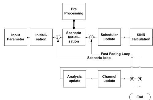
Bild 7 Blockschaubild des System-Level Simulators
