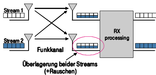
Bild 4 Prinzip des räumlichen Multiplexing (Single User MIMO)
