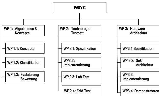
Bild 2 EASY-C Projektstruktur
